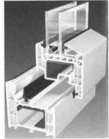
Schockline-Exklusiv-Fenster werden im Rahmen und Flügel mit einer Bautiefe von 73 mm gefertigt.
